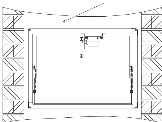
Вентиляционная шахта
